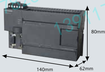
CPU 224XP CN / 224XPsi CN (14DI / 10DO + 2AI / 1AO)
